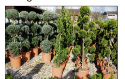
Formgehölze
